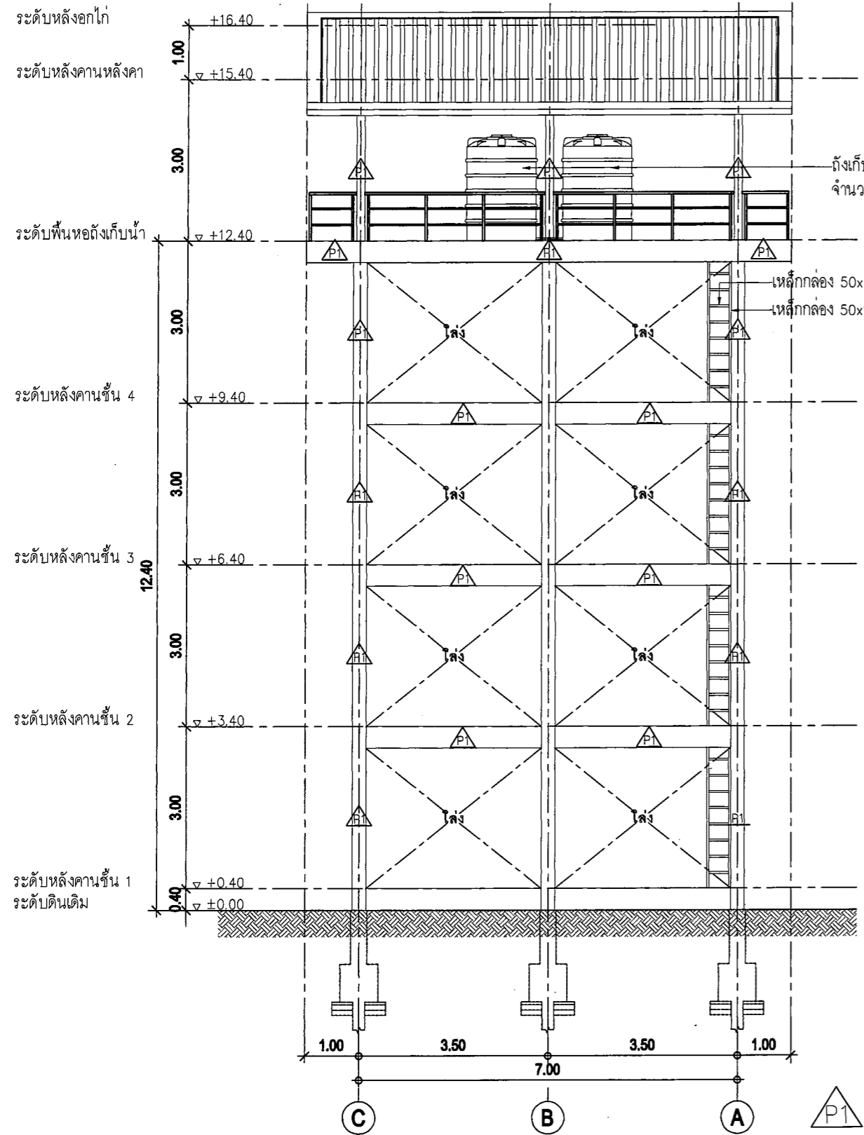
แบบรูปด้าน 3 มาตรฐาน 1 : 100
