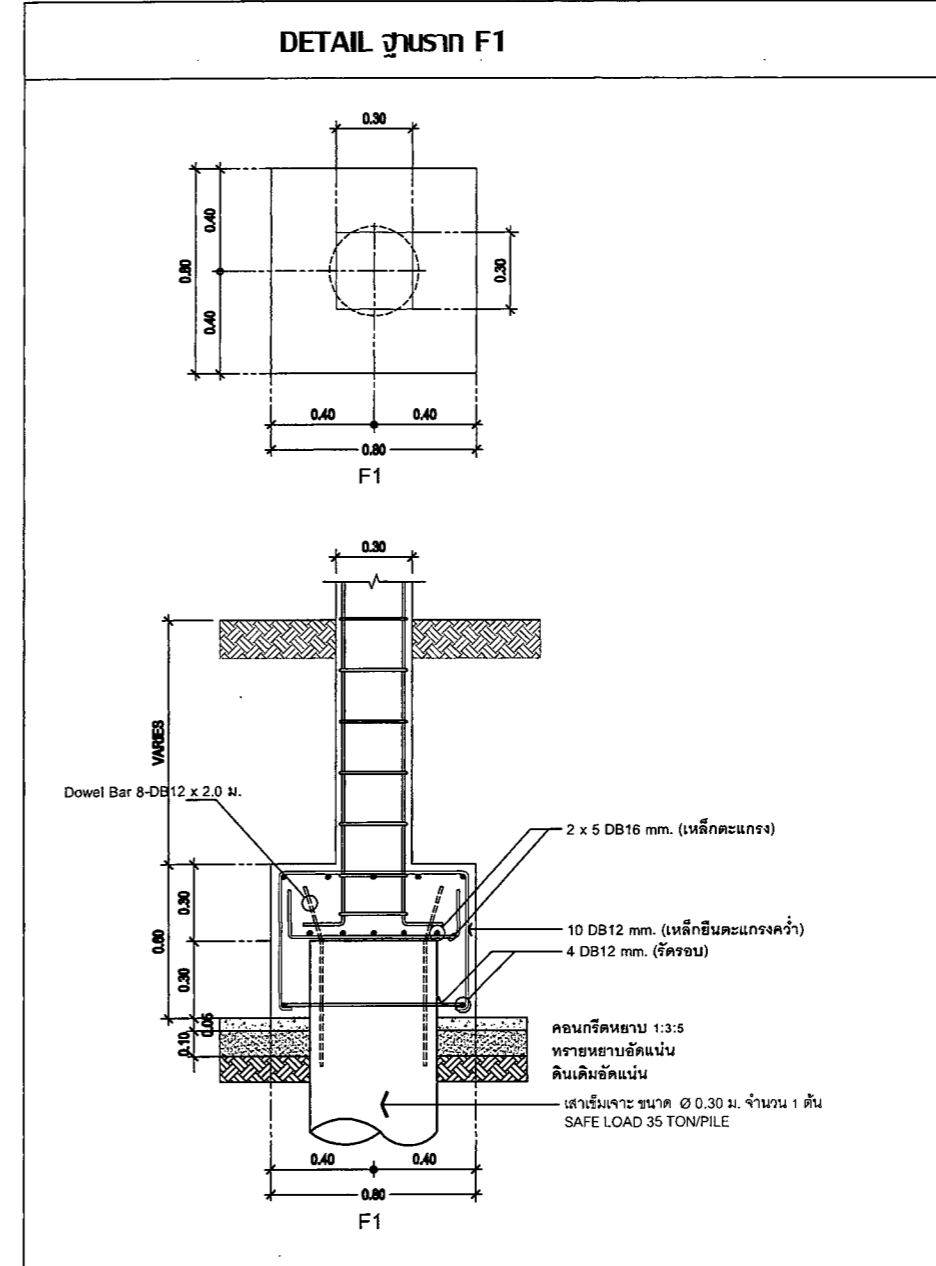
แบบขยายฐานราก มาตรฐาน 1 : 100
