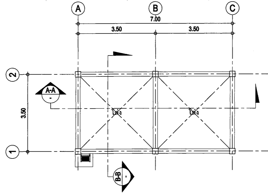
แบบแปลนพื้น ชั้นที่ 2,3,4
