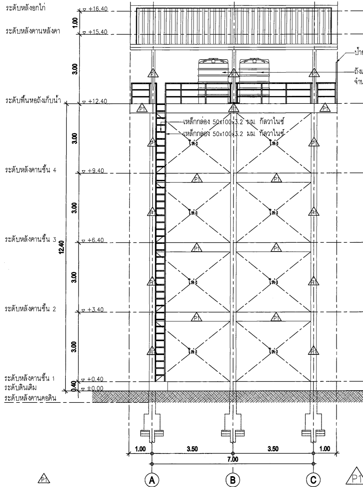
แบบรูปด้าน 1 มาตรฐาน 1 : 100
