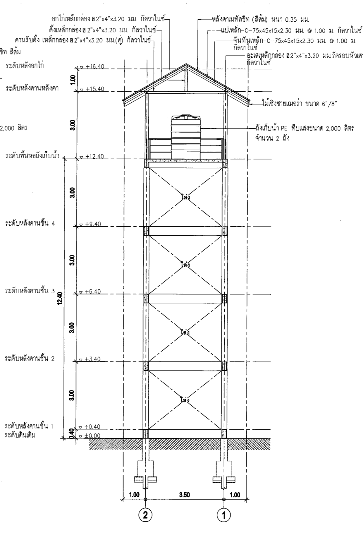
แบบรูปตัด B-B มาตรฐาน 1 : 100
