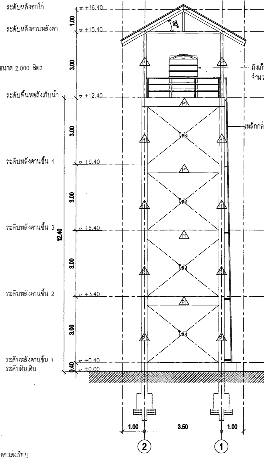
แบบรูปด้าน 2 มาตรฐาน 1 : 100
