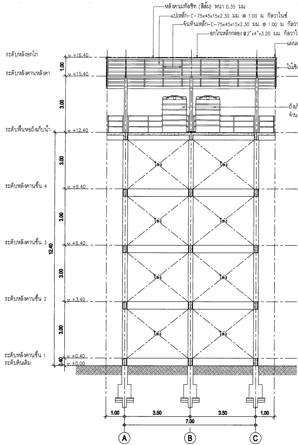
แบบรูปตัด A-A มาตรฐาน 1 : 100
