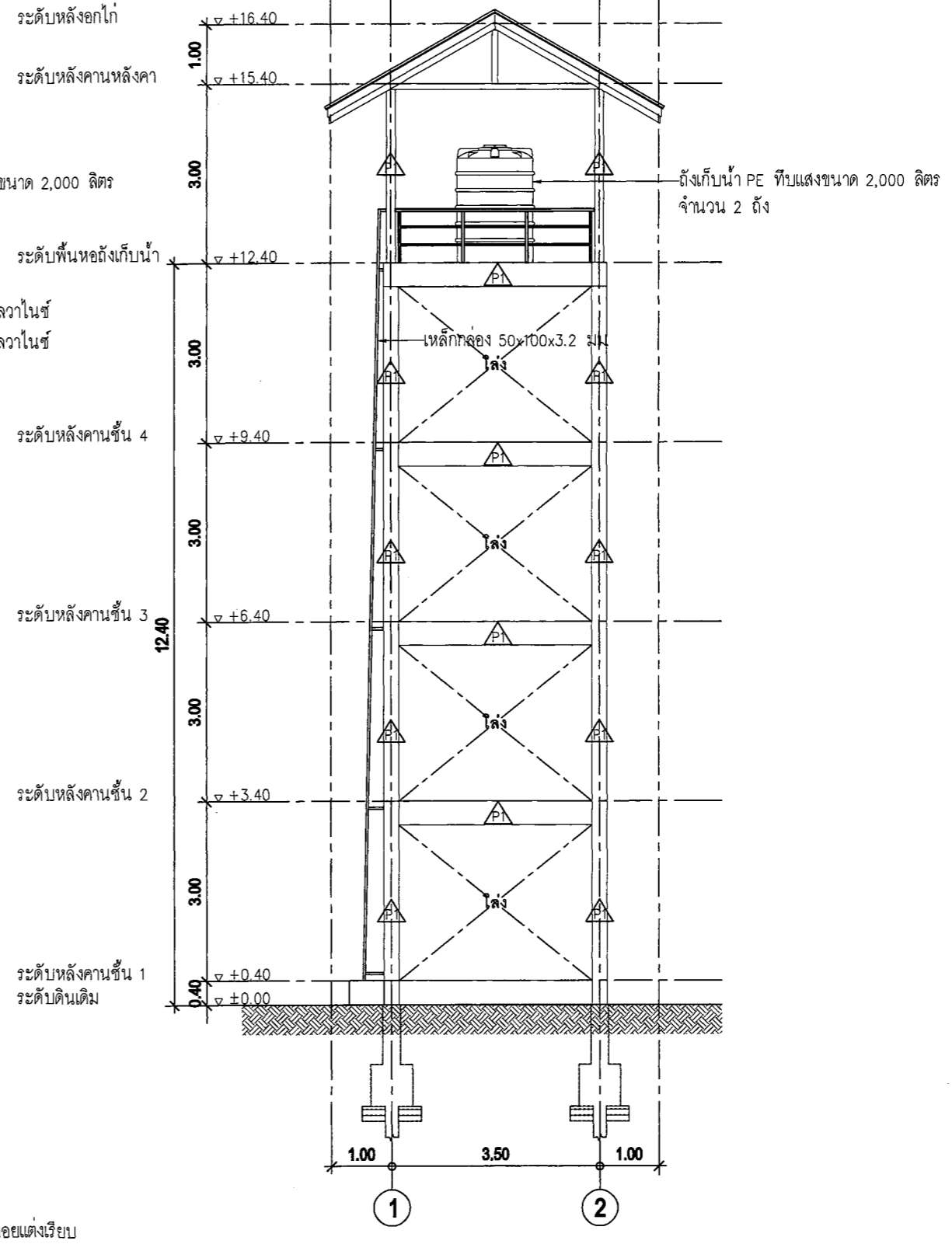
แบบรูปด้าน 4 มาตรฐาน 1 : 100
