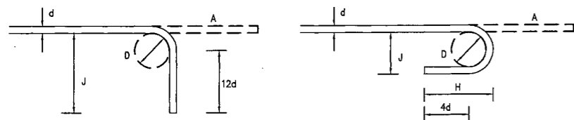
การงอขอ 90°
