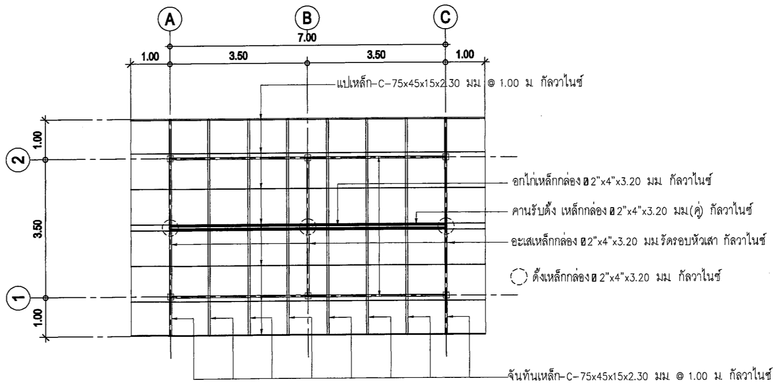
แปลนโครงเหล็กหลังคา มาตรฐาน 1 : 100
